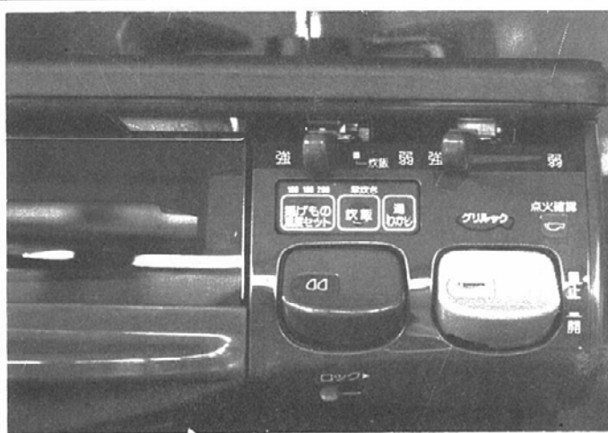
揚げ物の自動調温160℃180℃200℃、炊飯、湯沸の各ボタン
